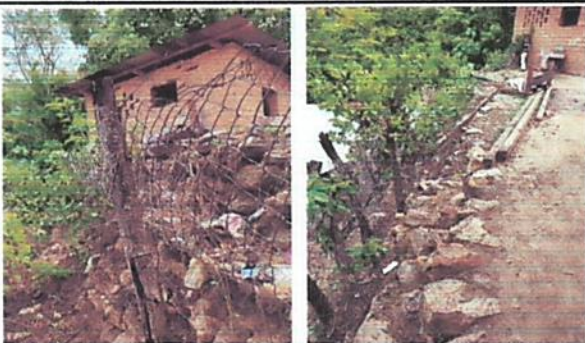
FOTO 5: MALLA EN MAL ESTADO Y LOS NIÑOS PELIGRAN CAER
